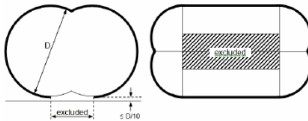
Tanques bilobulares
