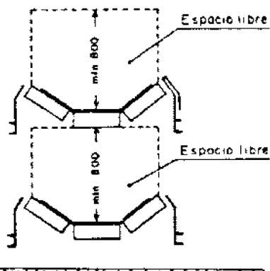
Fig. 6b. Transporte de personal en el ramal superior e inferior. Gálibos
