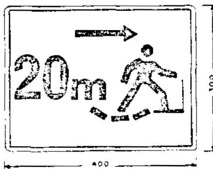
Fig. 8a. Indicador de estación de bajada a 20 m y sentido de salida de la cinta
