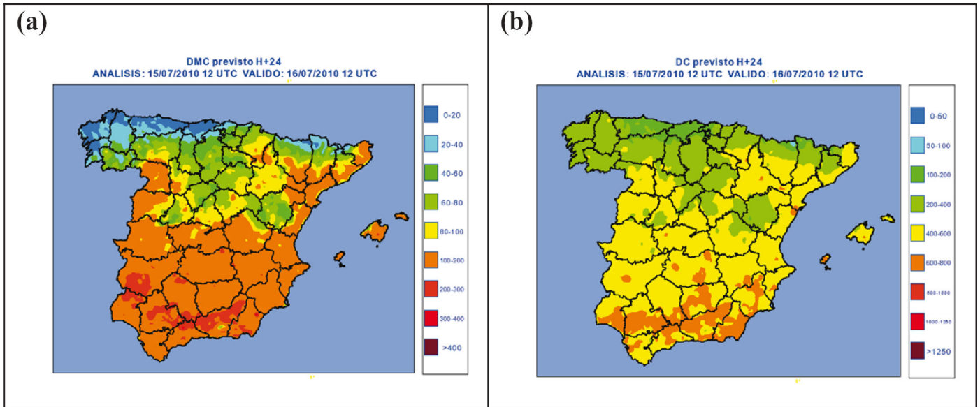
Fig. 33. Mapas previstos H + 24 del: (a) Subíndice DMC; (b) Subíndice DC.
