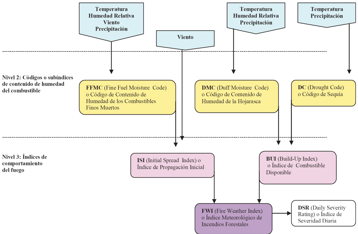
Fig.1. Estructura del Sistema FWI y orden secuencial en el cálculo del índice FWI
